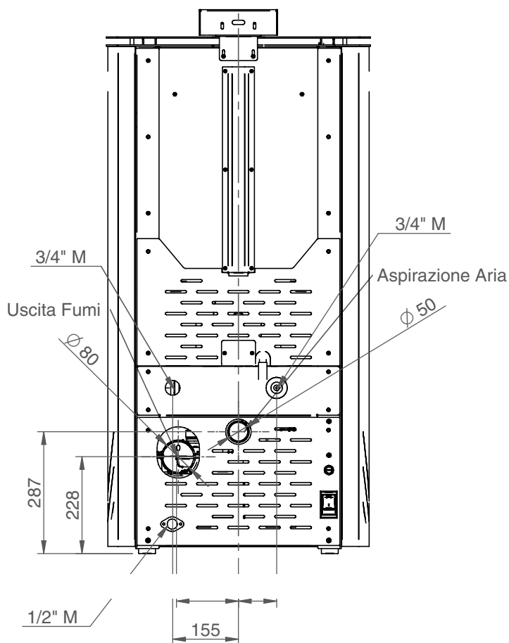
CONFIGURAZIONE STANDARD
