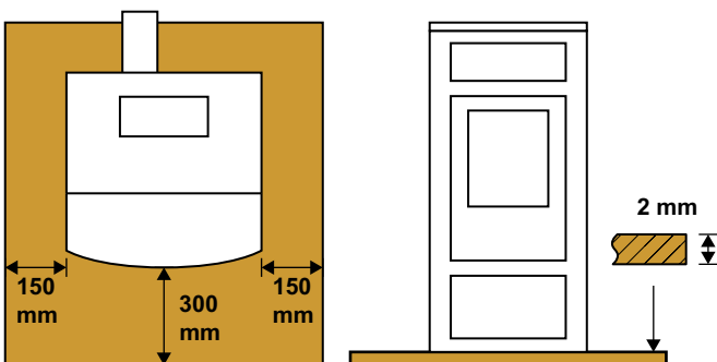
Piastra salvapavimento
