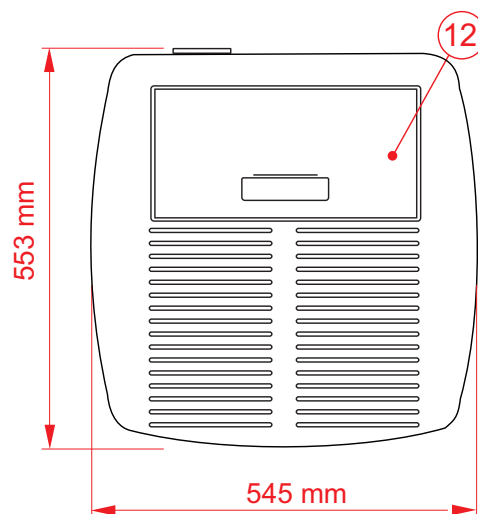
Vue supérieure
