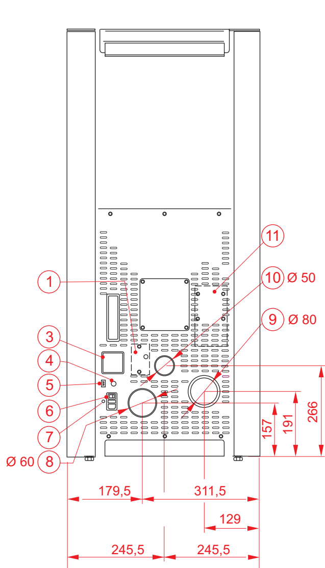
Vista posteriore
