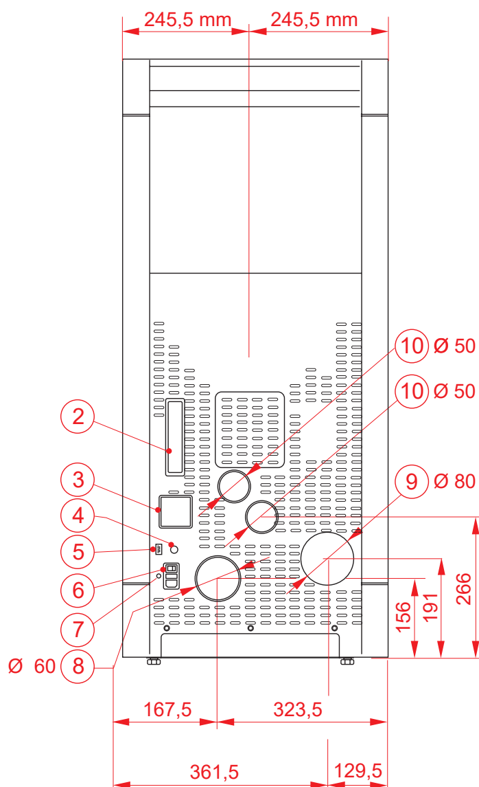
Vista posteriore
