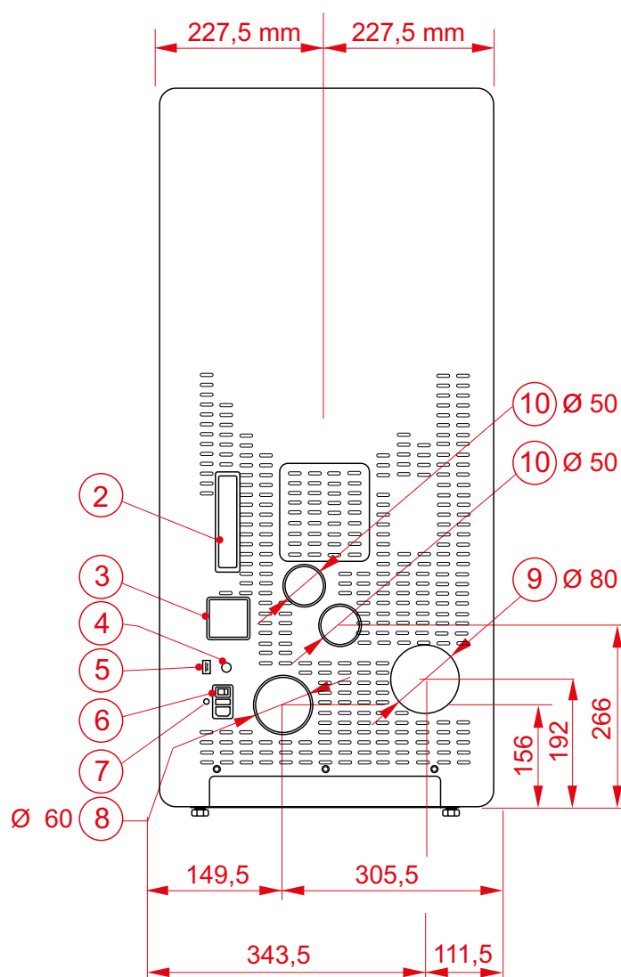
Vista posteriore
