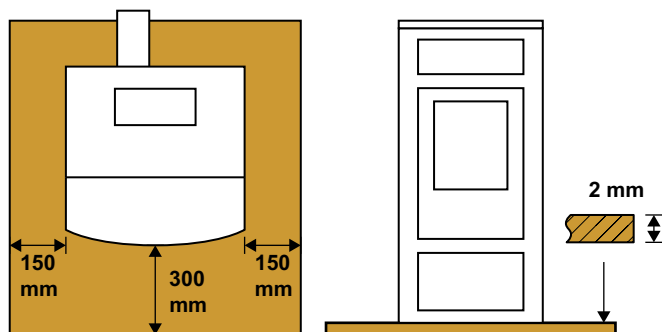
Piastra salvapavimento
