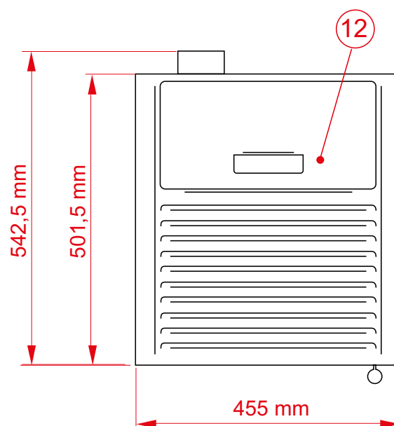
Vista superiore
