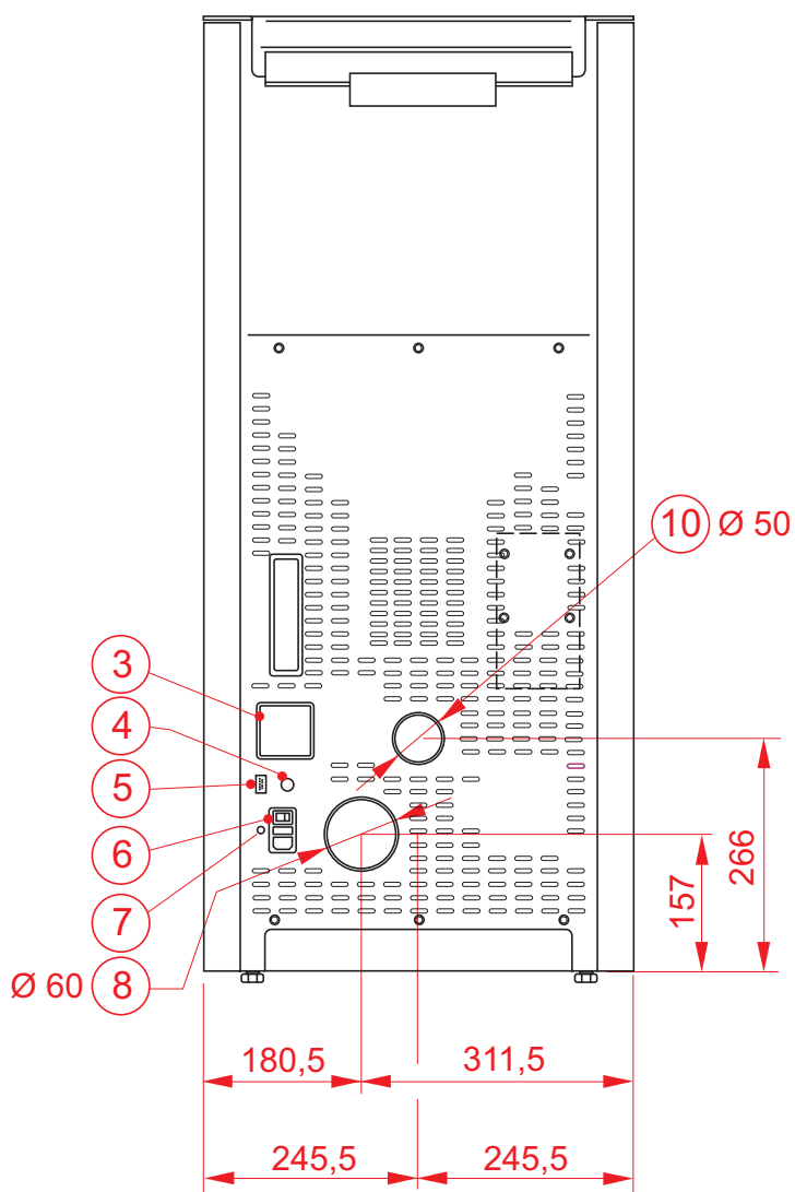
Vista posteriore
