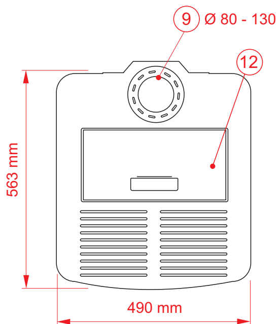
Vista superiore
