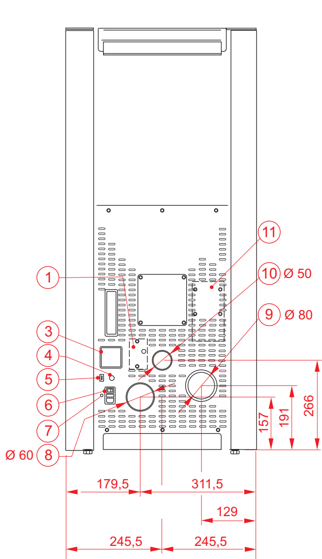
Vista posteriore
