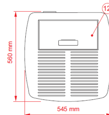
Vista superiore
