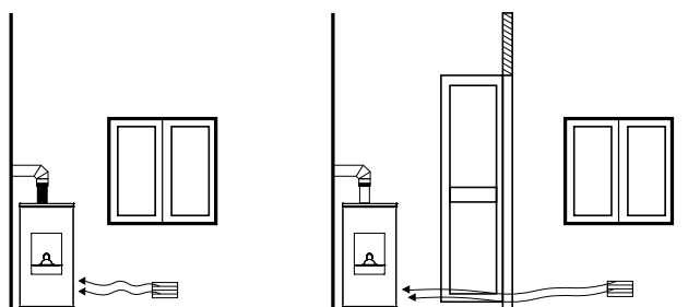
Fig.1a - DIRETTAMENTE DALL'ESTERNO Fig.1b - PER VIA INDIRECTA DAL LOCALE ADIACENTE
